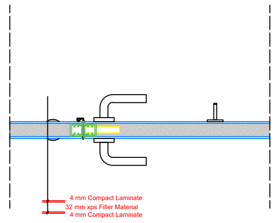
A-A SECTION
